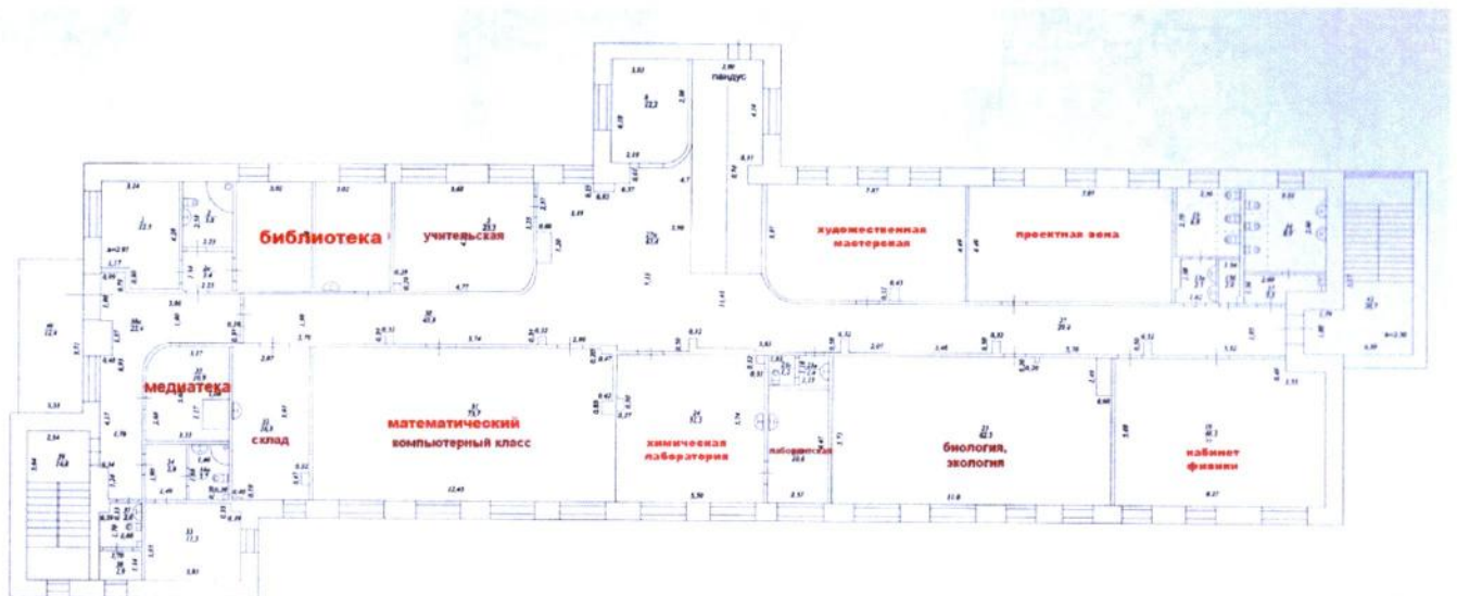
Рис.2. Зонирование. Учебный корпус № 1, 2-й этаж. Площадь – 660,4 кв.метра.
